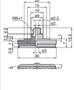
VP4x30E[5]-M6[9] 質量：2.8g[3.5g]
