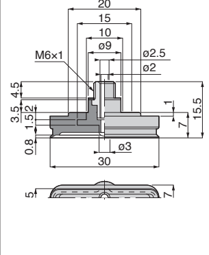
VP5x30E[5]-M6[9] 質量：2.8g[3.4g]
