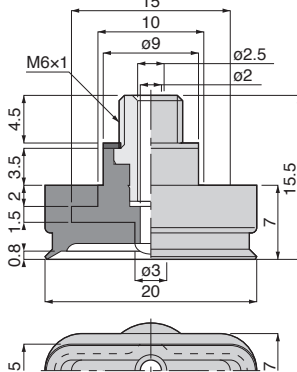
VP5x20E[5]-M6[9] 質量：2.4g[2.8g]
