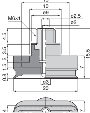
VP4x20E[5]-M6[9] 質量：2.4g[2.8g]
